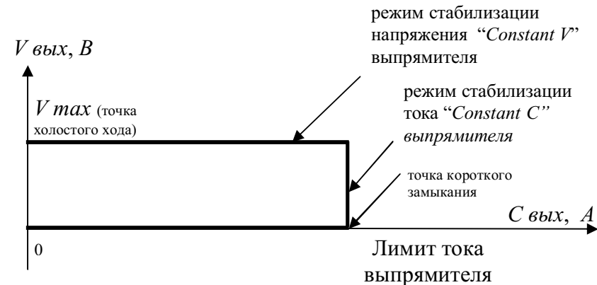
Рис. 14 Вольт-амперная характеристика работы выпрямителя
