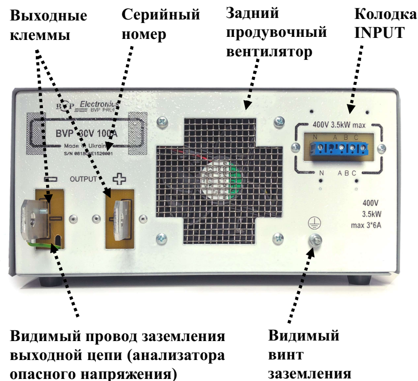
Рис. 6. Внешний вид задней панели силового модуля
