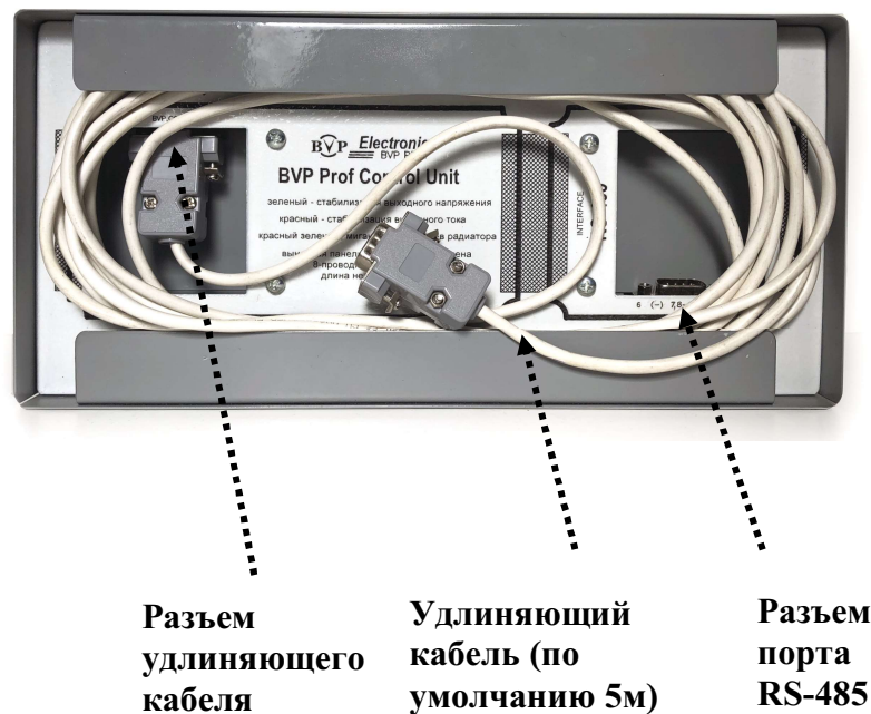
Рис. 4. Внешний вид задней части пульта управления
