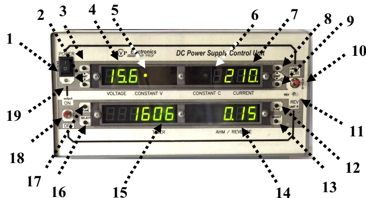
Рис. 3. Расположение органов управления на лицевой части пульта управления
