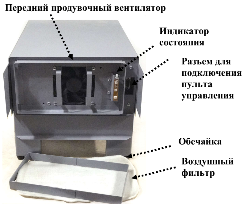
Рис. 5. Передняя панель силового модуля без фильтра
