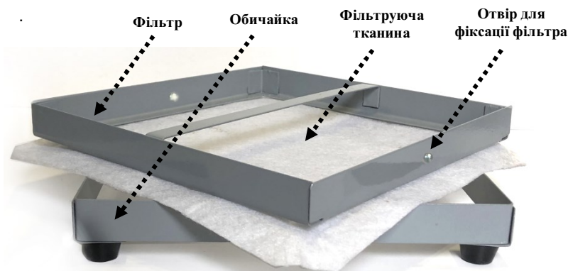
Мал. 5. Знімний повітряний фільтр
