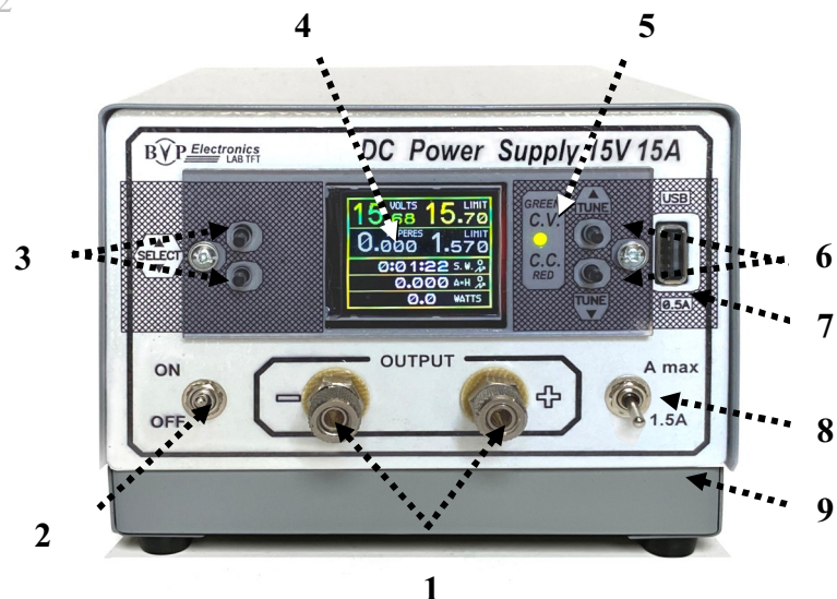
Рис. 2. Расположение органов управления на передней панели источника питания
