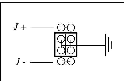
Рис. 11 Снятие заземления с выходных клемм источника
