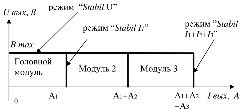
Рис. 6 Вольт-амперная характеристики при параллельном подключении модулей
