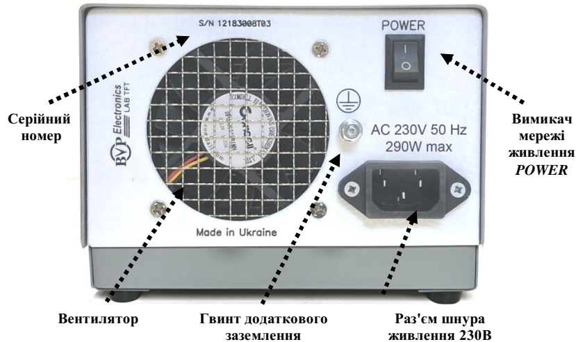
Мал. 4. Розташування органів управління на задній панелі джерела живлення
